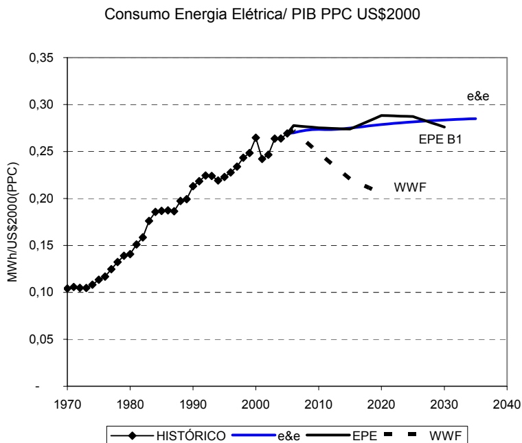
Figura 5.5: Simulação do consumo de energia elétrica da EPE com o programa da e&e e da WWF alterando-se o parâmetro de participação futura da energia elétrica no consumo total. Esta aproximação deu origem aos valores revistos da Tabela 5.1
